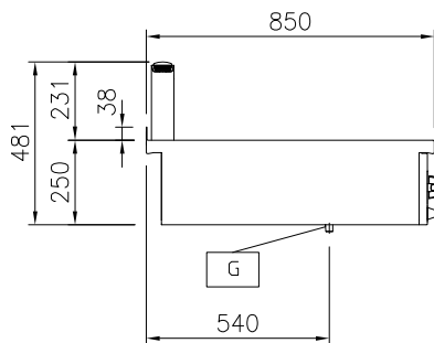
Zij aanzicht
